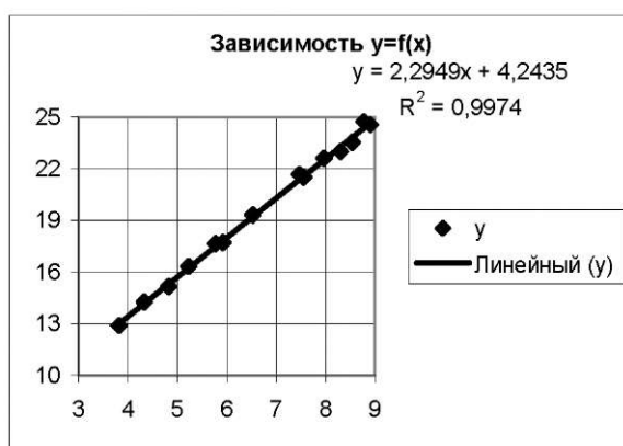
Рисунок 2.1 – Пример диаграммы с уравнением зависимости
