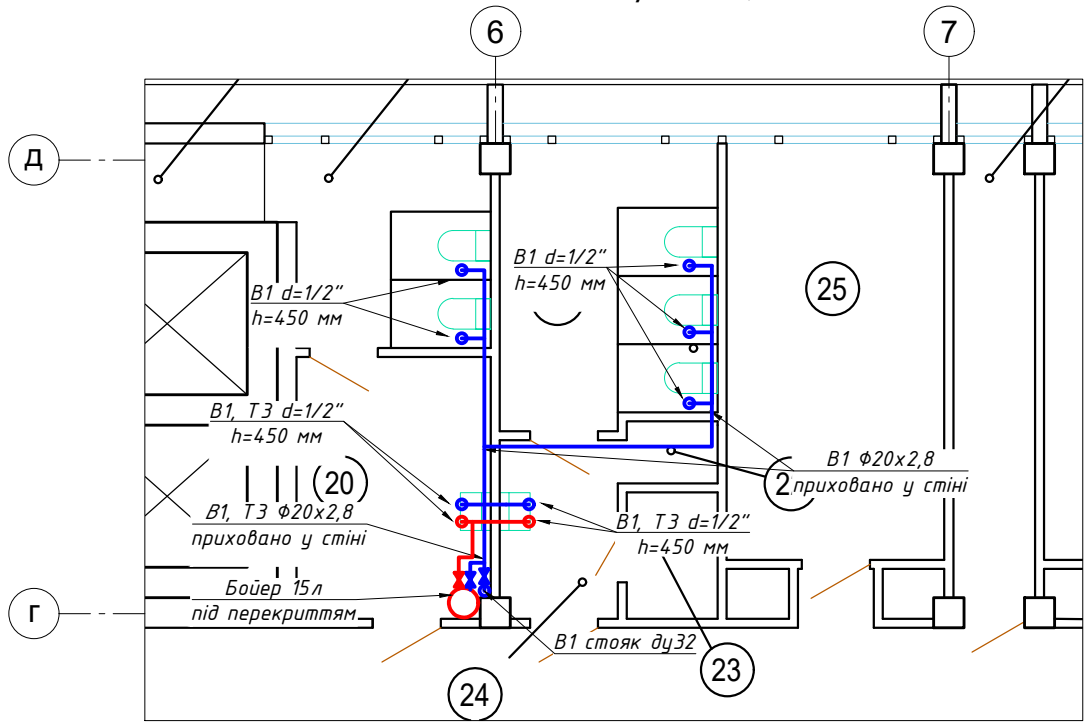
Санвузол 7-го поверху в осях 6-7/Г-Д Мережі В1, Т3 Т4
