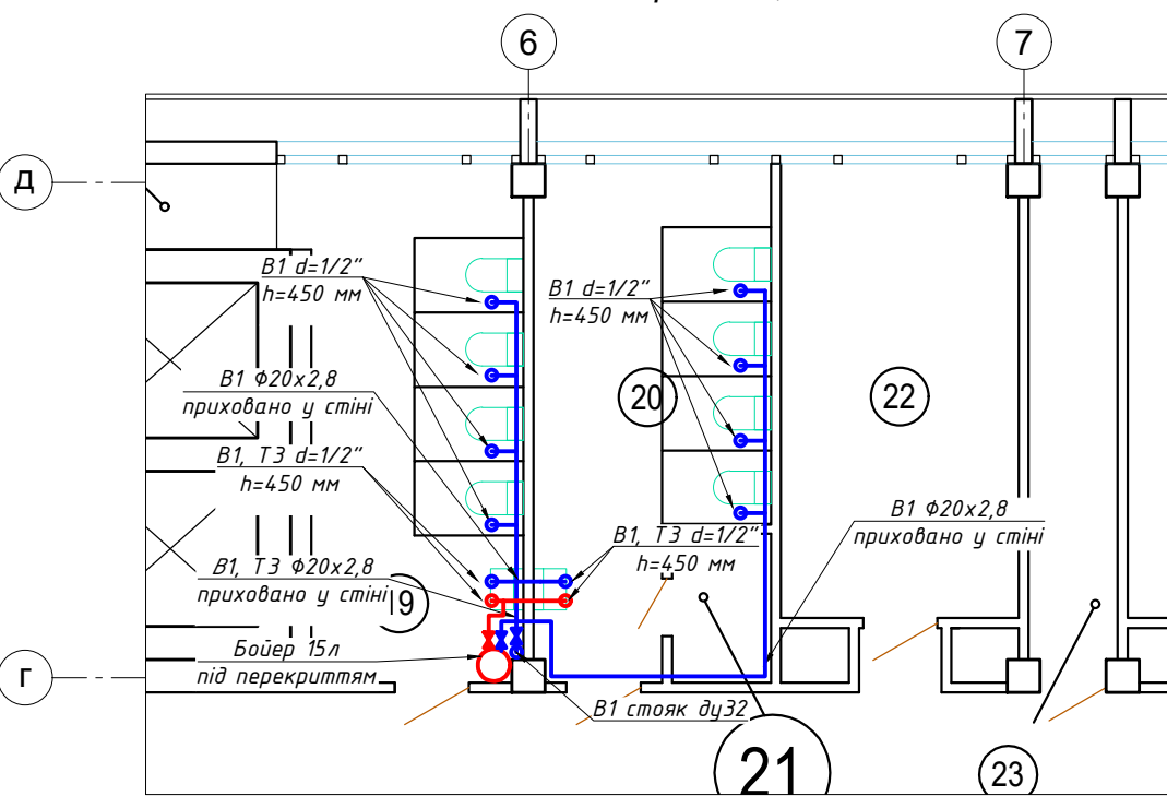
Санвузол 6-го поверху в осях 6-7/Г-Д Мережі В1, Т3 Т4
