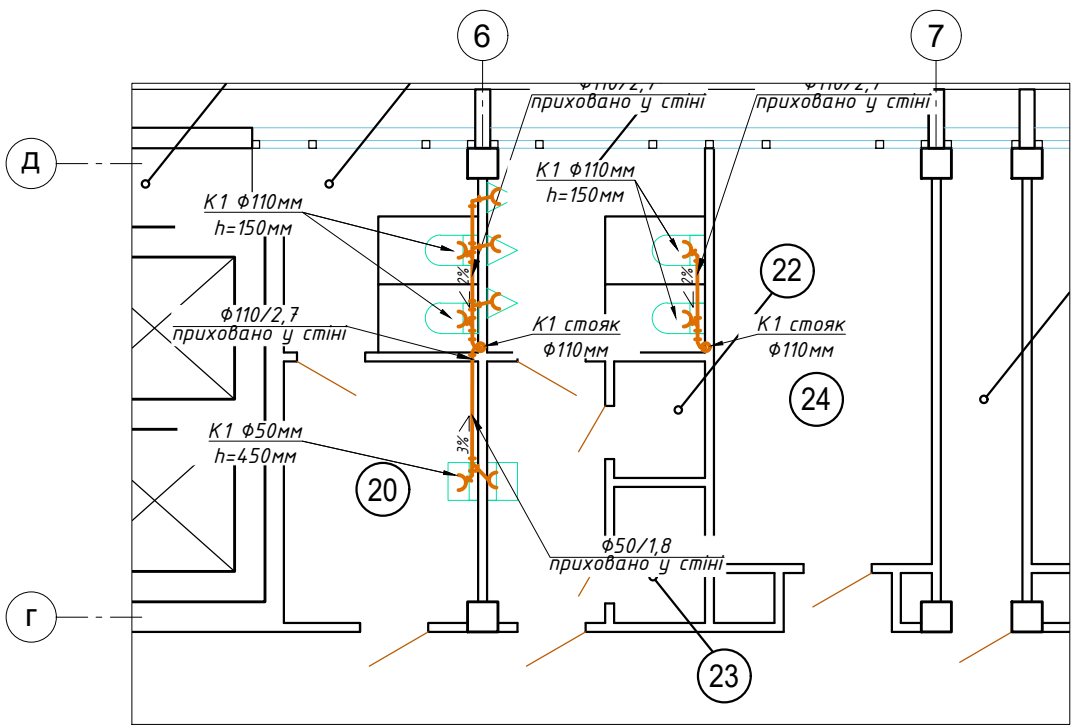
Санвузол 5-го поверху в осях 6-7/Г-Д Мережі К1
