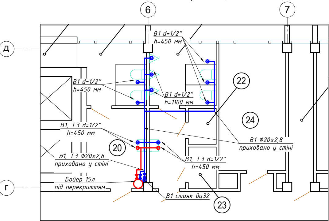
Санвузол 5-го поверху в осях 6-7/Г-Д Мережі В1, Т3 Т4
