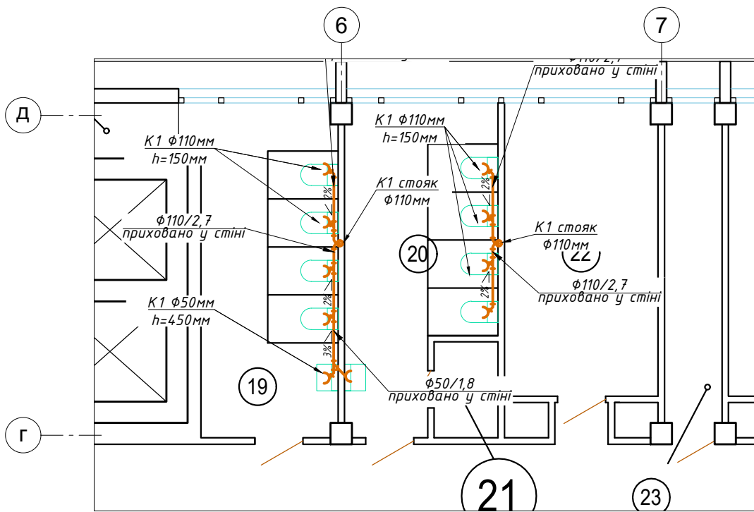
Санвузол 6-го поверху в осях 6-7/Г-Д Мережі К1
