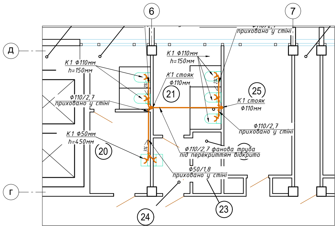
Санвузол 7-го поверху в осях 6-7/Г-Д Мережі К1
