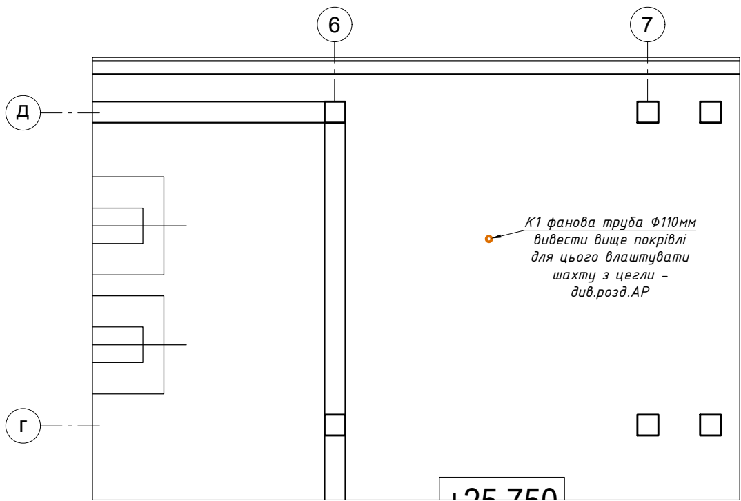
Технічний поверх в осях 6-7/Г-Д Мережі К1
